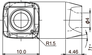
Fig.2 SPET100415ZPER-SM
