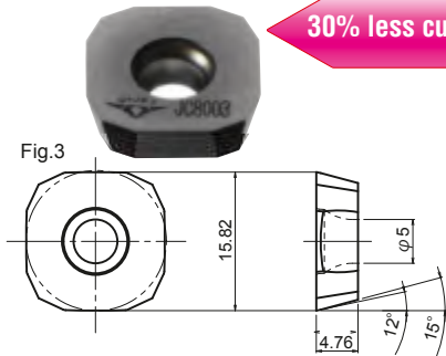
SDHW1504ADEN-F1
