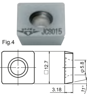
SPHW1203ZPTR
