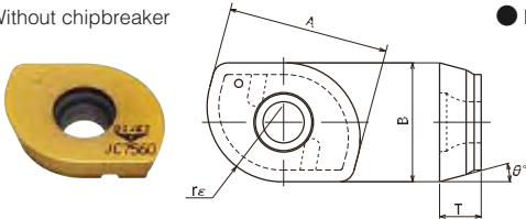
● Fig 1. Without chipbreaker
